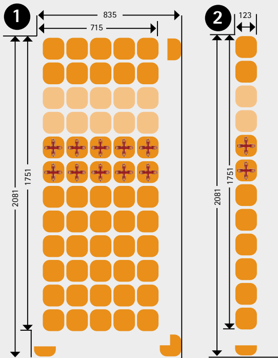
1 Grundpaket Basic bed kit 2 Erweiterungspaket Expansion package
